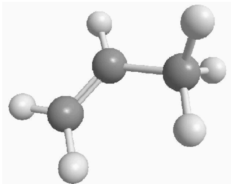
Figure 2 : La molécule de propylène. Les atomes de carbone sont représentés par des sphères gris foncés, ceux d'hydrogène par des sphères gris clair. Cliquer sur l'image pour l'agrandir
