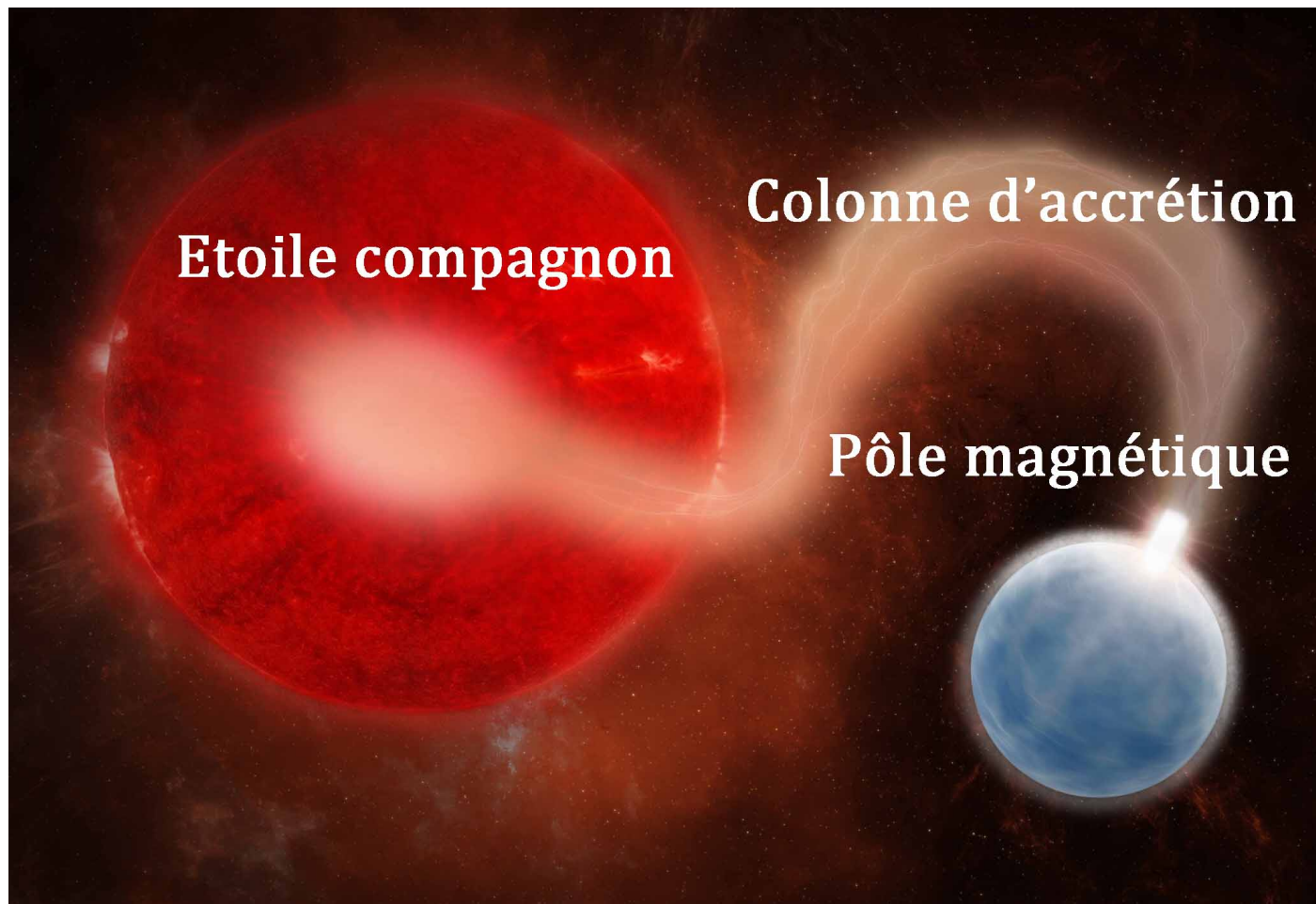
Schéma de l'attraction de matière exercée par une naine blanche (à droite) sur une étoile voisine (à gauche). La matière « aspirée » forme une colonne d'accrétion, qui se concentre au niveau du pôle magnétique de la naine blanche. © Animea/F. Durillon
