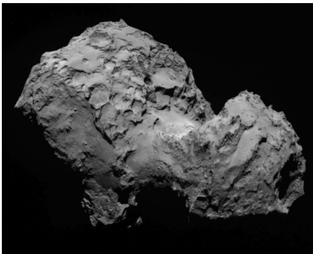
Le noyau de la comète « Tchouri » (Churyumov-Gerasimenko) observé par la sonde européenne Rosetta. © ESA/Rosetta/MPS for OSIRIS Team MPS/UPD/LAM/IAA/SSO/INTA/UPM/DASP/IDA
